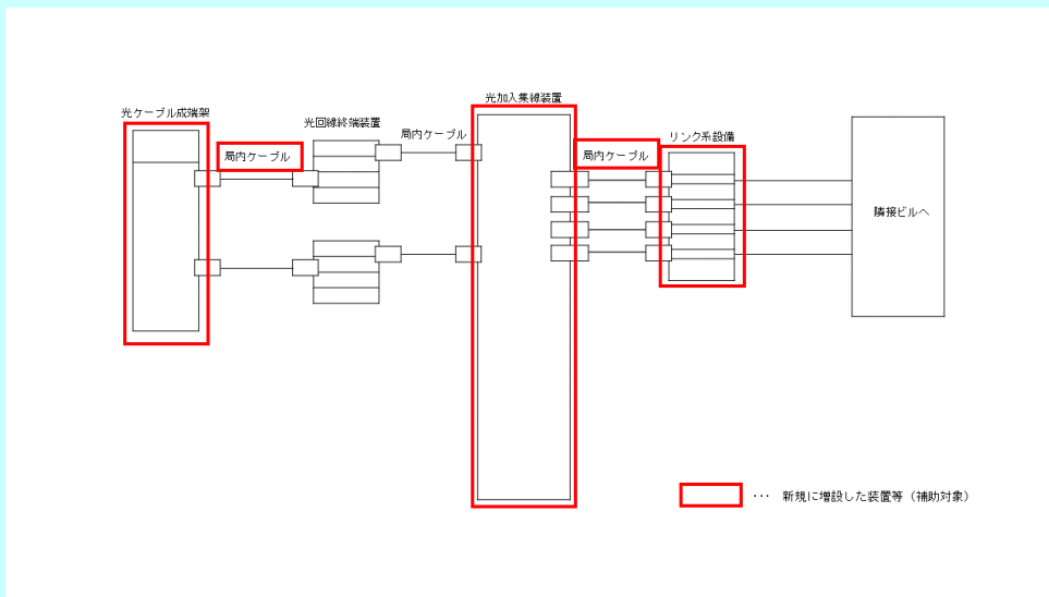
【装置系統図（例）】
