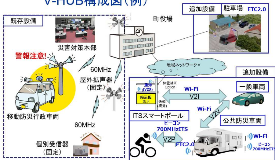
図2 V-HUB の構成図 (例)
