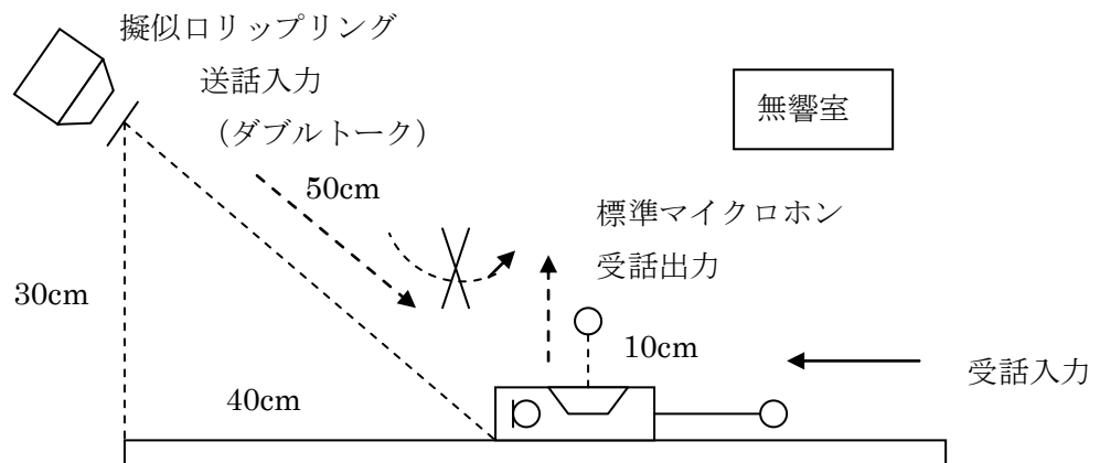
図7 受話挿入損失の測定
