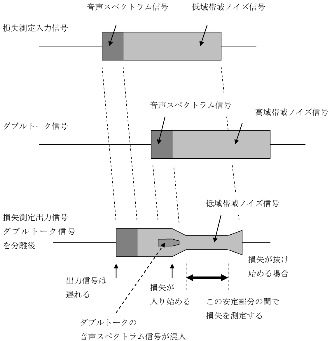
図14 挿入損失の測定
