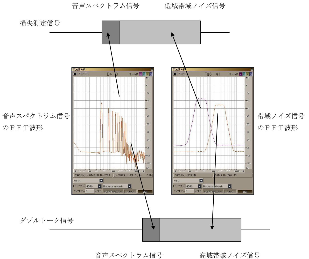
図10 測定信号とダブルトーク信号の分離
